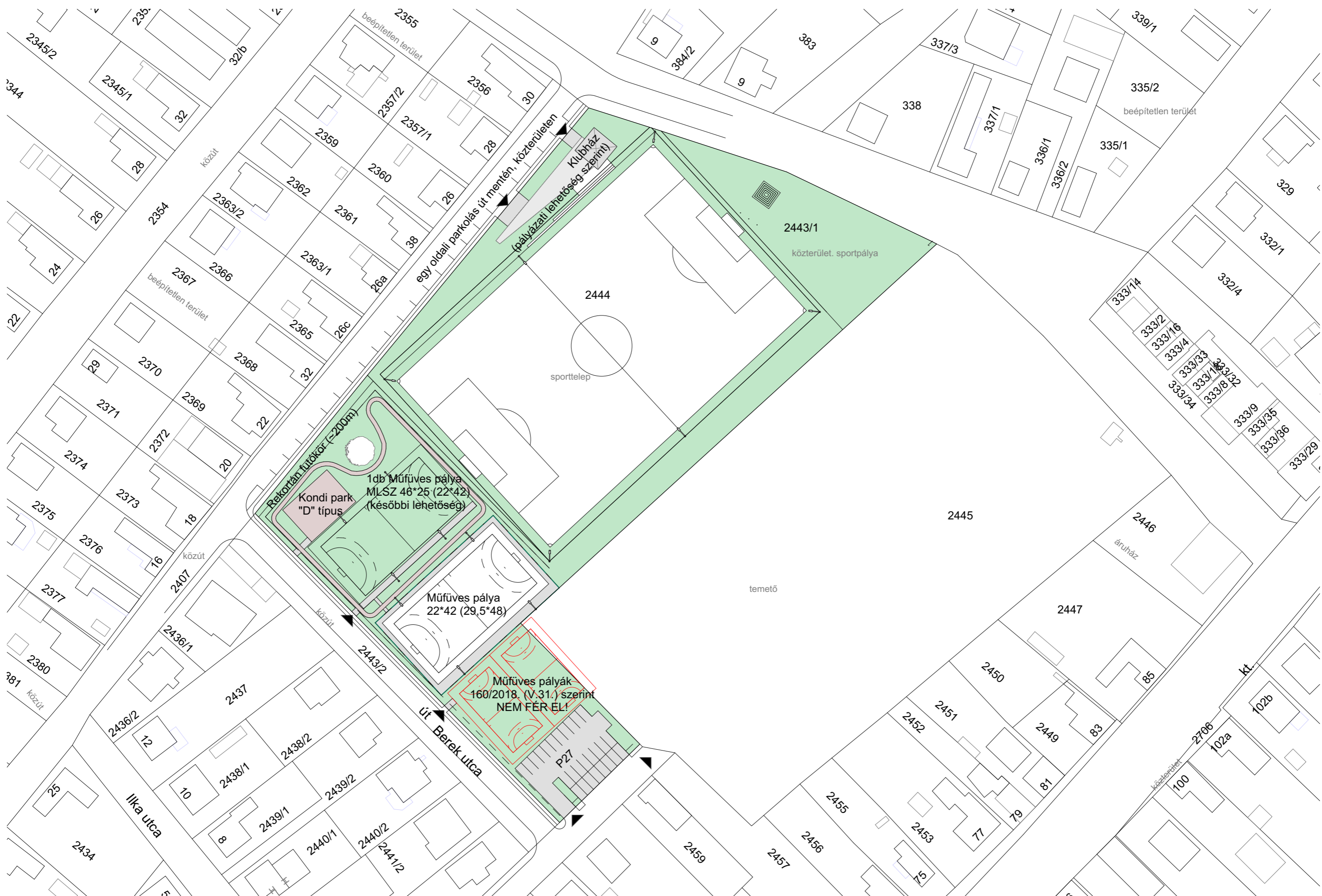
Kerepes, Jelenlegi sporttelep fejlesztési helyszínrajza M=1:1000
