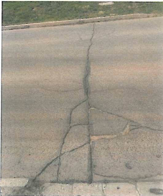
Hálós repedések az útburkolaton
